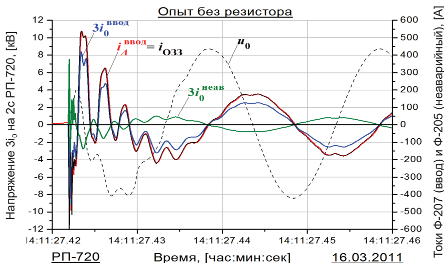
Рис. 1. Опыт металлического однофазного замыкания на землю
