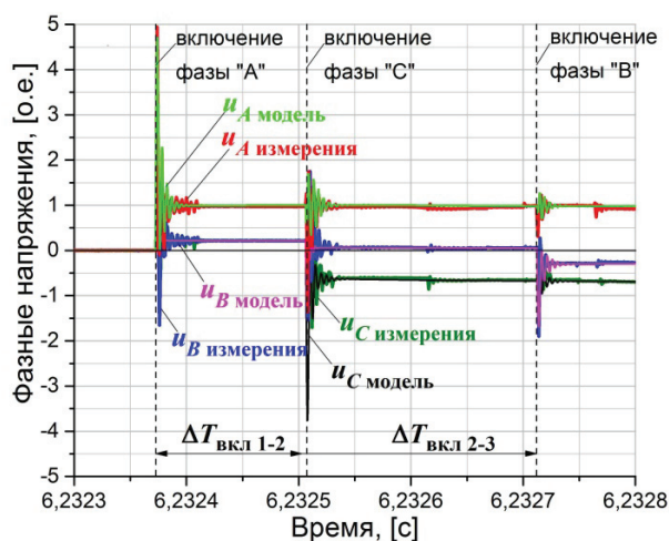
Рис. 3. Сопоставление результатов экспериментальных измерений с результатами математического моделирования
