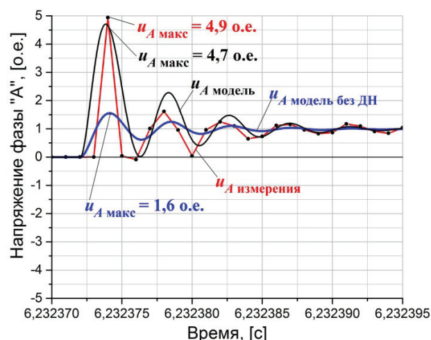
Рис. 3. Сопоставление результатов экспериментальных измерений с результатами математического моделирования
