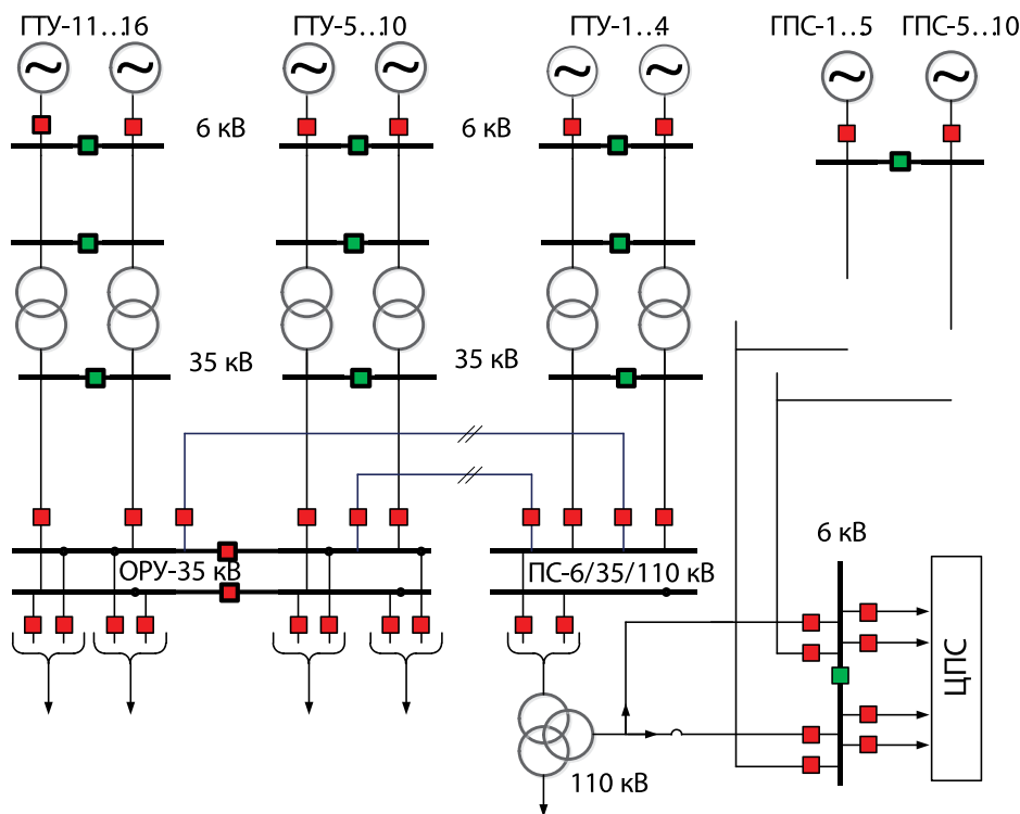
Рис. 1. Приведенная схема энергосистемы месторождения
