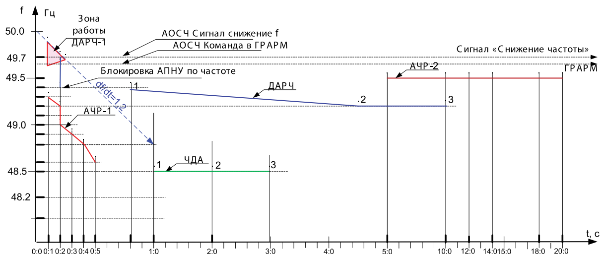
Рис. 2. Диаграмма селективности
