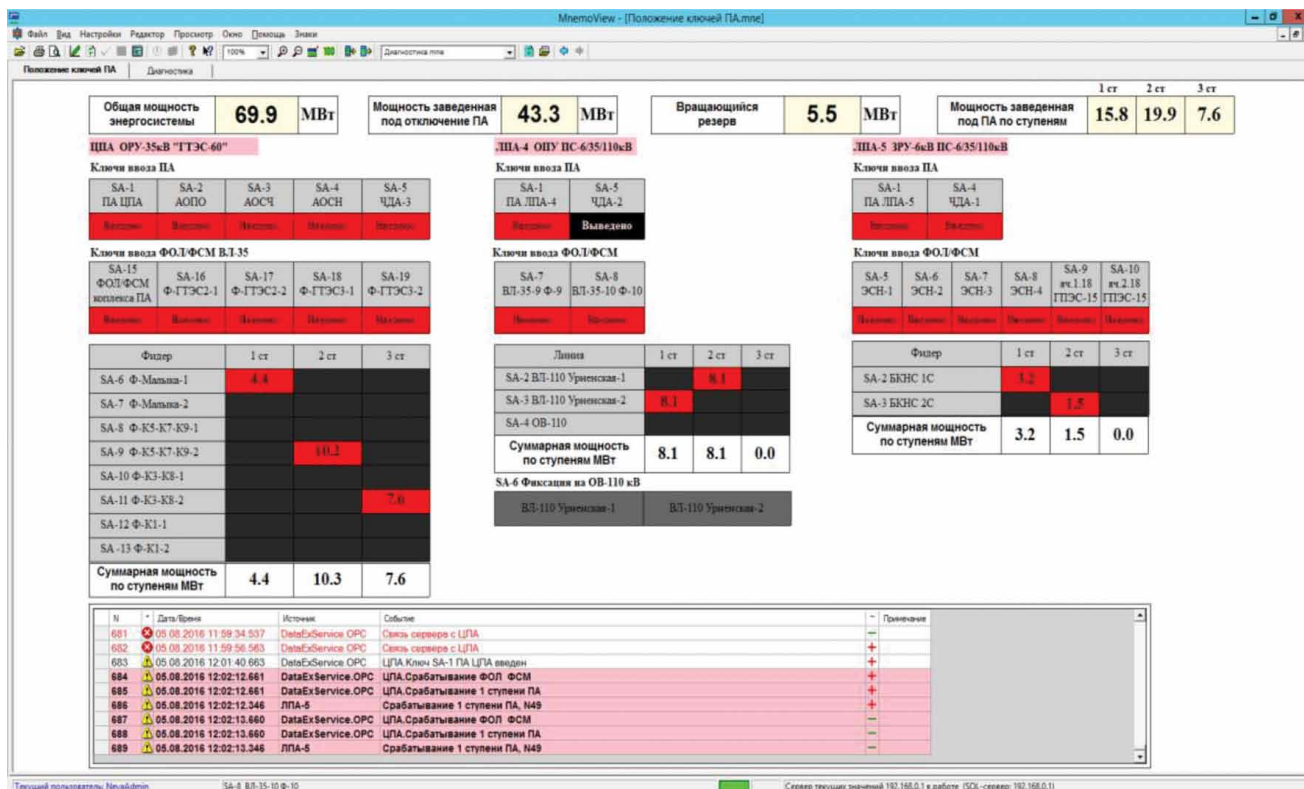
Рис. 4. Видеограмма ПА объекта
