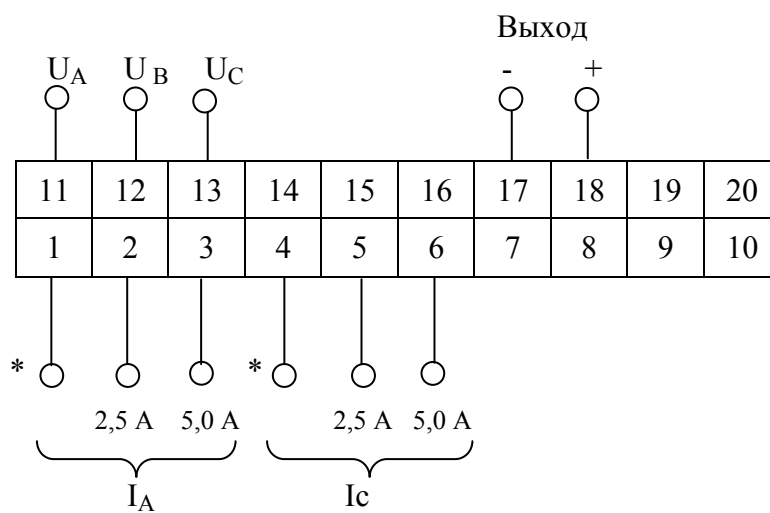
Рисунок А.3 – Схема подключения ИП Е 860/1ЭС, Е 860/3ЭС, Е 860/6ЭС
