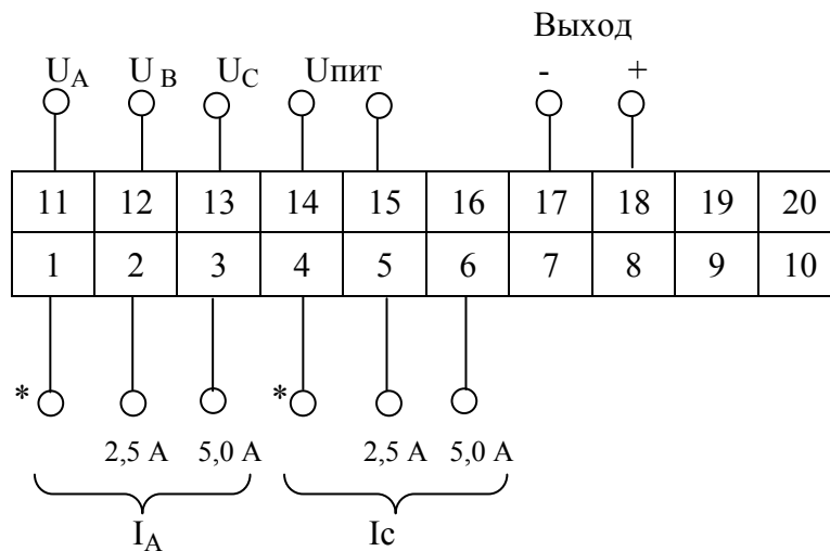
Рисунок А.2 – Схема подключения ИП Е 860/2ЭС, Е 860/4ЭС, Е 860/5ЭС
